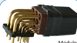
Module à picots coudés femelle
