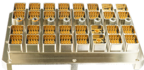
Platines métalliques SIM / EN4165 (exemple avec modules SIM équipés de contacts à sertir normalisés avec protection or)
