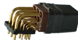
Module à picots coudés femelle Female module with angled PCB contacts
