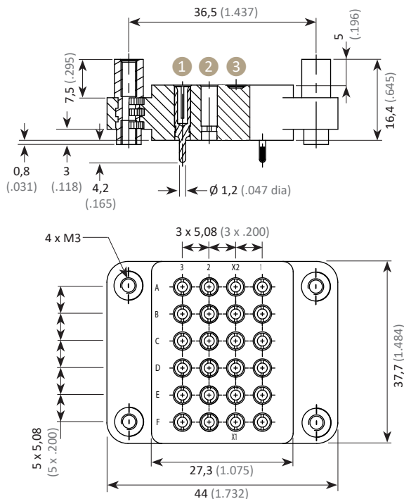
Dimensions avec colonnettes non détrompées Dimensions with not polarized pillars
