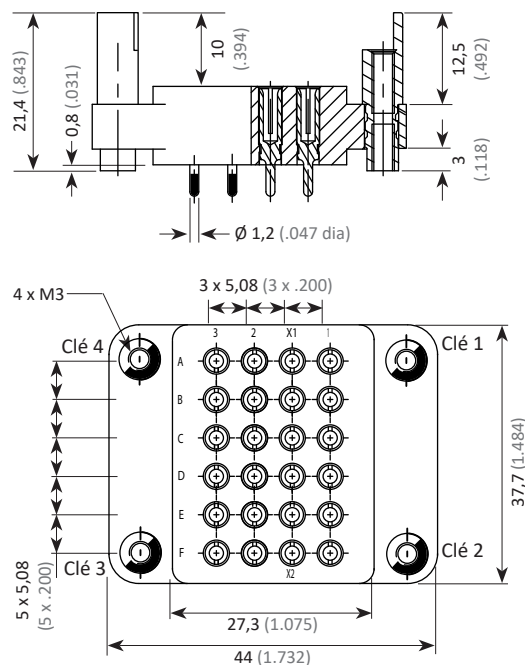
Dimensions avec colonnettes détrompées Dimensions with polarized pillars
